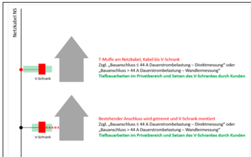
Abbildung 4: Fall 1: V-Schrankmontage an Längskabel, Fall 2: V-Schrankmontage an vorhandenen Netzanschluss (eigene Darstellung)
