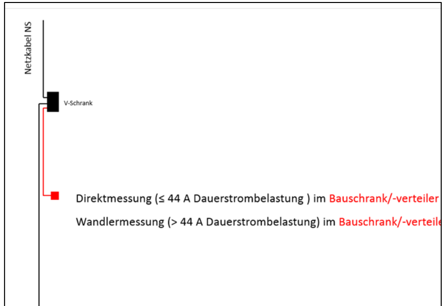
Abbildung 1: Anschluss an Kabelverteilerschrank (eigene Darstellung)
