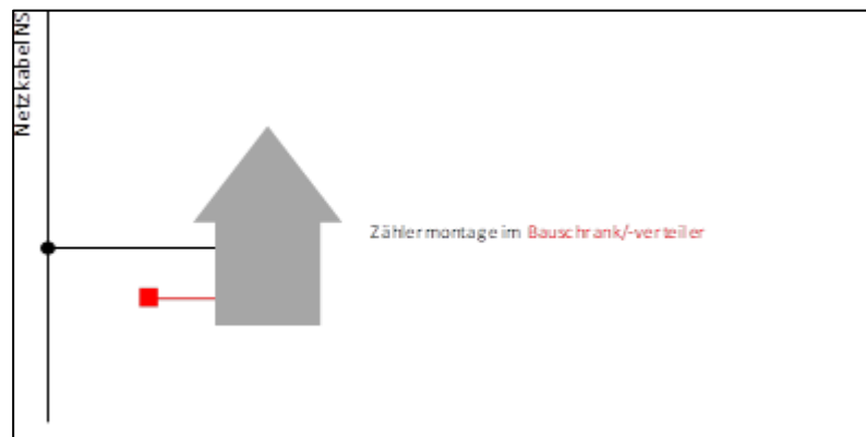
Abbildung 2: Anschluss an Zähleranlage Nachbarhaus (eigene Darstellung)
